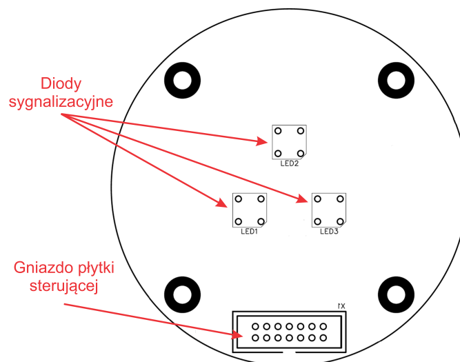
Rysunek 10: Rzut na kluczowe elementy elektroniczne płytki sygnalizacyjnej
